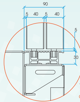
ДЕТАЛЬ -А МАСШТАБ 1:5 A : تفصيلات DETAY A ÖLÇEK 1:5 مقياس: 1:5
