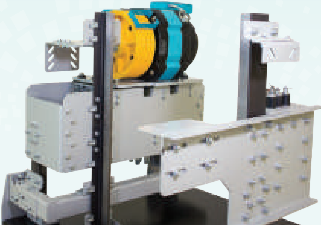
2:1 Askı Karkaslar 2:1 Acting Car Frames Каркас с подвеской 2:1 إطارات نظام التعليق 1:2
