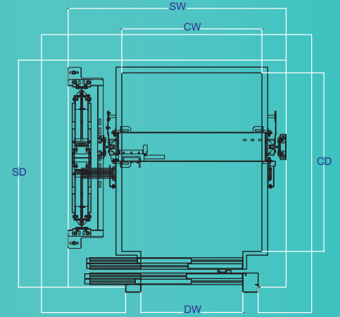
En Üst Kat Kesiti Last Floor Section Секция Верхнего Этажа نهاية على طابق
